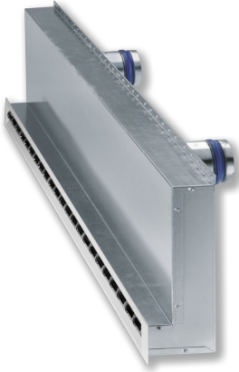
VSD50-1-LT-AZ-M-L/1175
